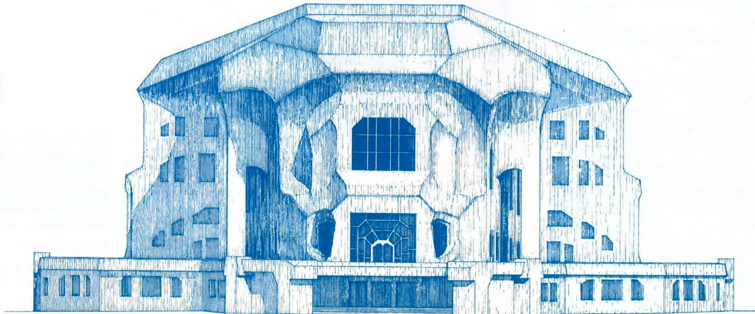
第二ゲーテアヌム 西立面図 上松祐二作画(1968)
